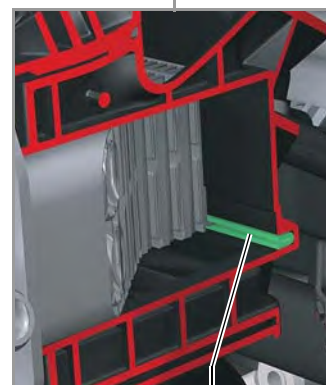
Уплотнительная пластина
