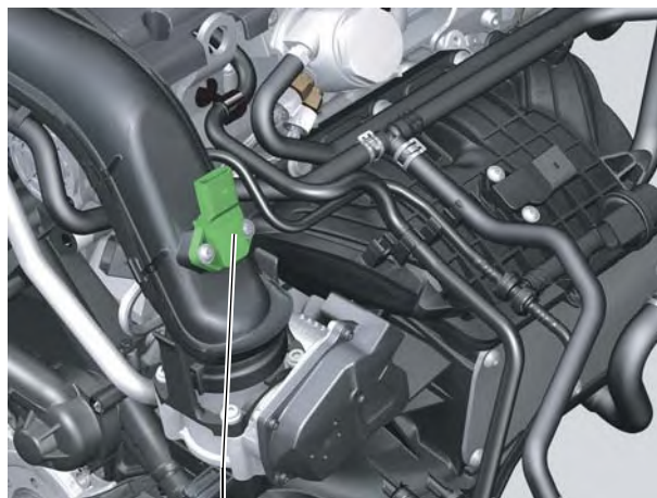
Датчик давления наддува G31 с датчиком температуры воздуха на впуске G299 S405_042
