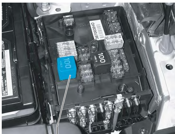
Реле дополнительного насоса системы охлаждения J496
