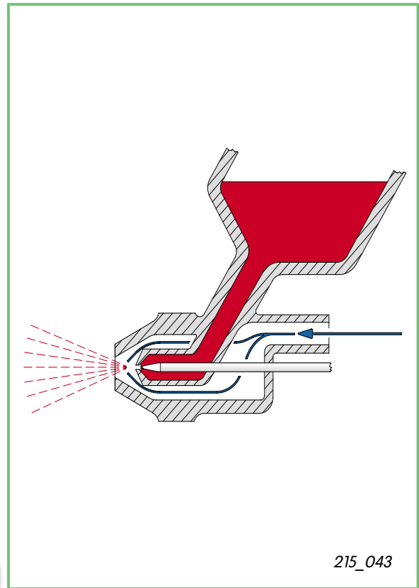
Jet pistol
